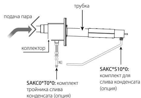
SAO* : отдельная горизонтальная трубка
