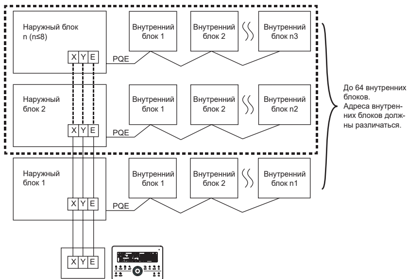
Центральный пульт управления, присоединенный к наружному блоку
