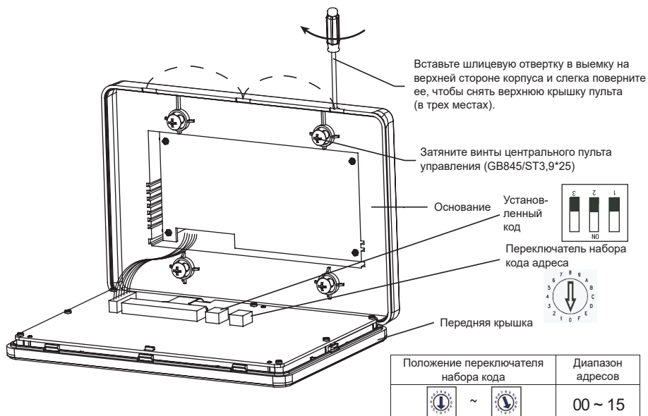
Рисунок 1.2. Монтажная схема
